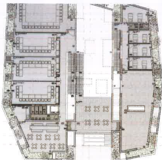
Plantas do piso 0 e piso 1 do edifício
